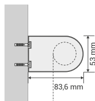
VISTA DI LATO Attacco a parete
